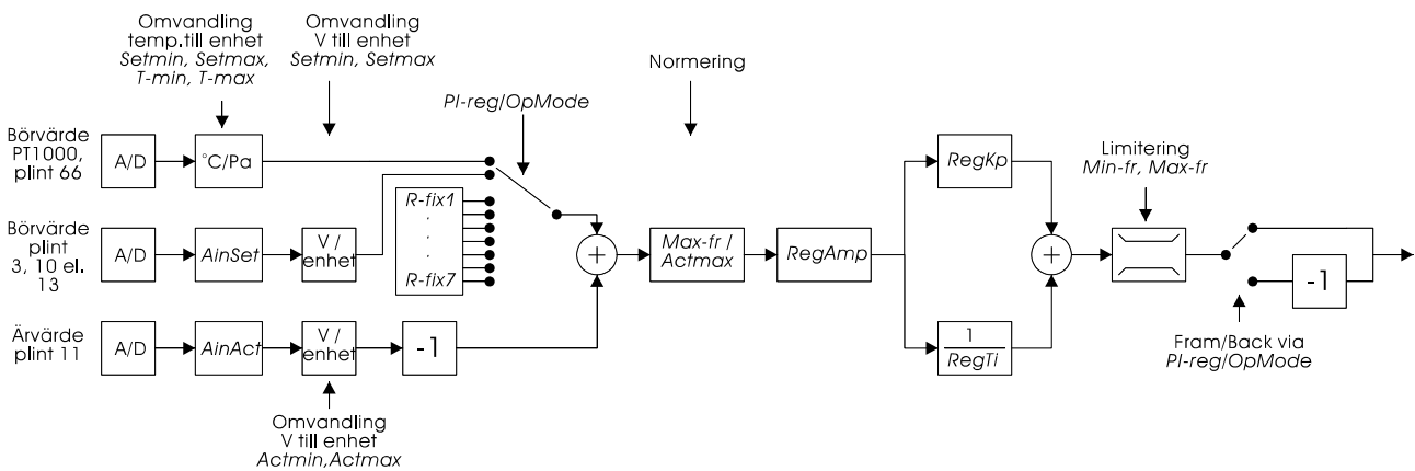
Figur 9. Översikt av processregulatorn
