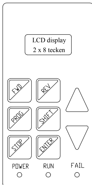
Figur 6. Tangentbordet
